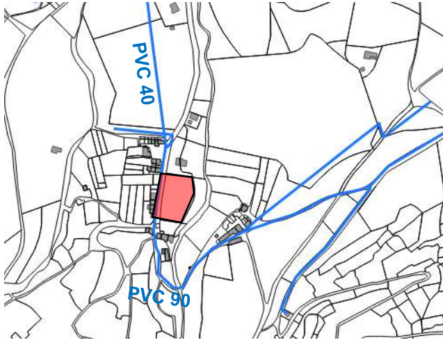
Réseau AEP
