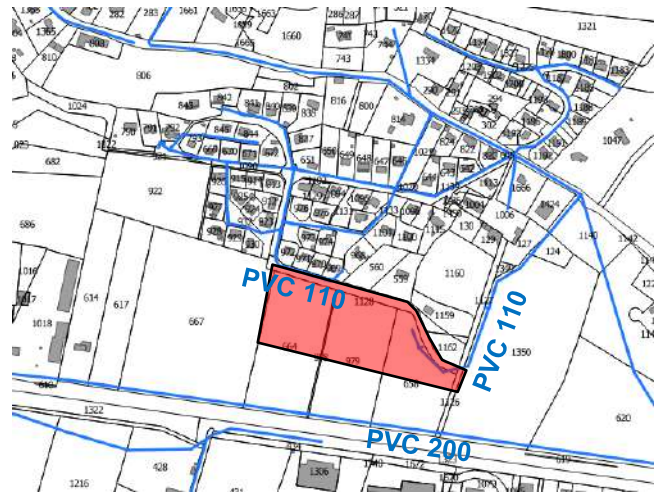
Réseau AEP
