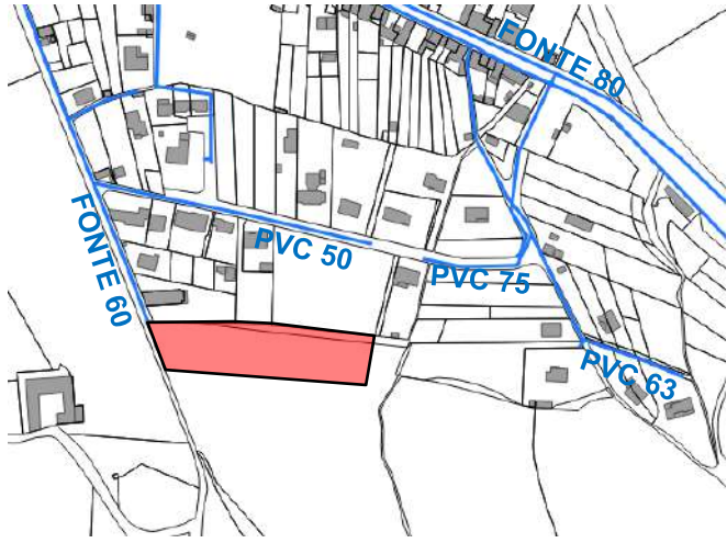
Réseau AEP
