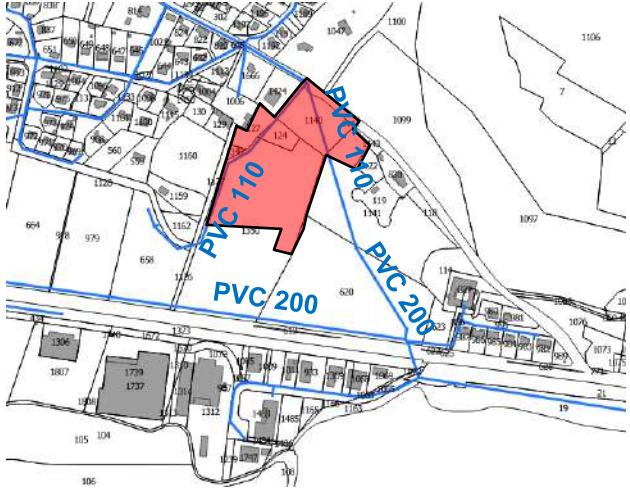
Réseau AEP
