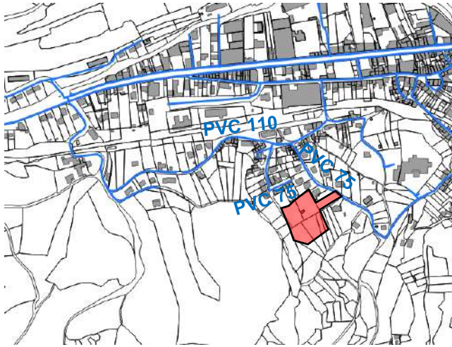
Réseau AEP
