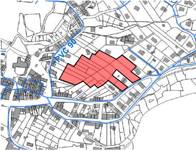
Réseau AEP
